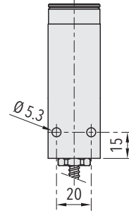
Stecker / Connecteur / Plug EN175301-803-A (DIN 43650-A) (Zubehör 58 / Accessoire 58 / Accessory 58)
